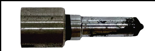
カーボンが付着したインジェクション
